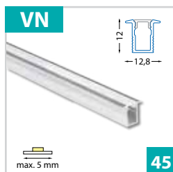
Vestavný hliníkový profil 13x12 mm - pro pásky do šíře 5 mm
