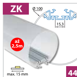
Závěsný hliníkový profil Ø 100 mm - pro pásky do šíře 15 mm
