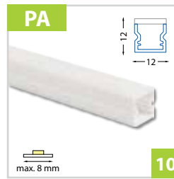
Přisazený PMMA profil 12x12 mm - pro pásy do šíře 8 mm
