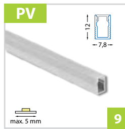
Přisazený hliníkový profil 8x12 mm - pro pásy do šíře 5 mm
