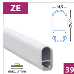
Závěsný hliníkový profil 15x30 mm - pro pásky do šíře 8 mm
