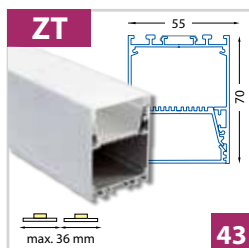
Závěsný hliníkový profil 55x70 mm - pro dva pásky do šíře 18 mm
