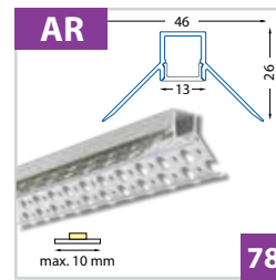
Rohový hliníkový profil pro sádkarton 46x26 mm - pro pásy do šíře 10 mm
