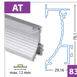
Vestavní hliníkový profil pro sádkarton 29x70 mm - pro pásy do šíře 12 mm
