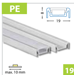
Přisazený hliníkový profil 19x8 mm - pro pásy do šíře 10 mm
