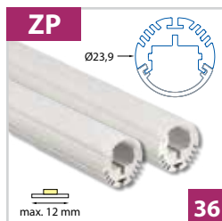
Závěsný kruhový hliníkový profil Ø 24 mm - pro pásky do šíře 12 mm
