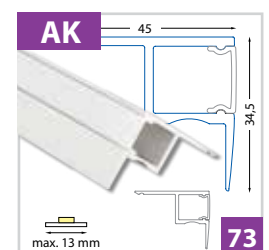
Podhledový hliníkový profil 45x35 mm - pro pásy do šíře 13 mm
