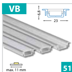
Vestavný hliníkový profil 23x7 mm - pro pásky do šíře 11 mm
