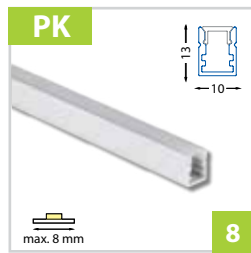
Přisazený hliníkový profil 10x13 mm - pro pásy do šíře 8 mm
