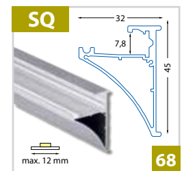
Speciální hliníkový profil, na sklo 8 mm - pro pásy do šíře 12 mm
